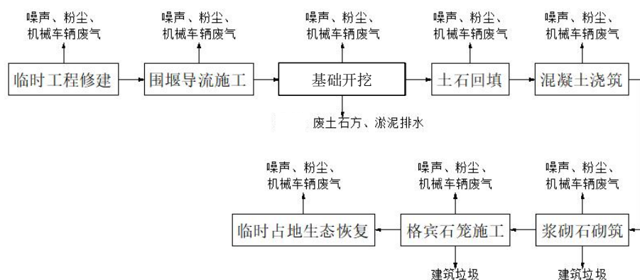
图4-1本工程施工期工艺流程及产污环节图
